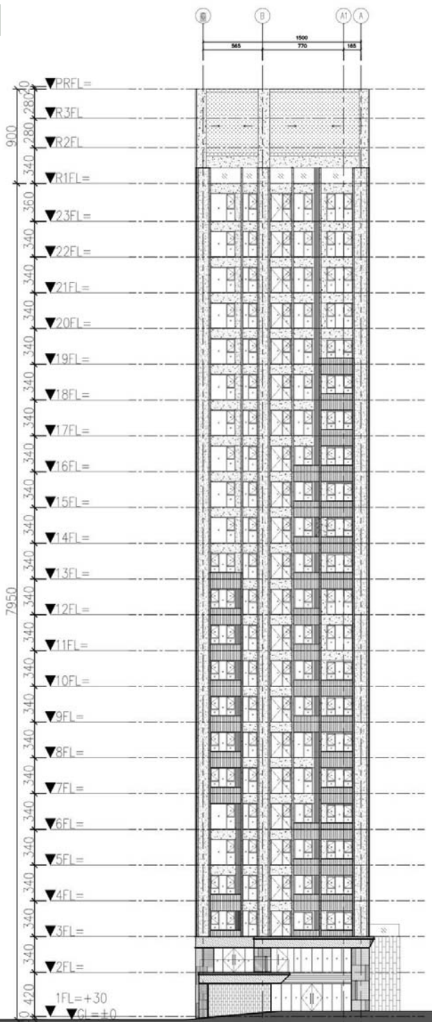
東向立面圖
